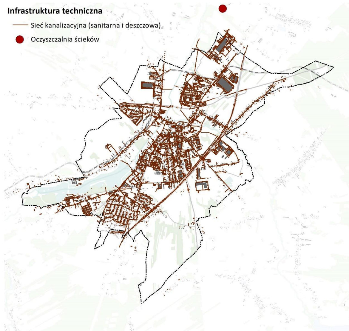
Rysunek 16. System sieci kanalizacyjnej w Rawie Mazowieckiej
