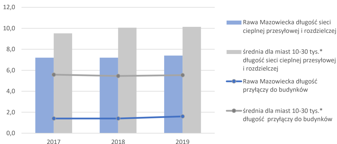
Wykres 82. Długość sieci ciepłowniczej przesyłowej i rozdzielczej oraz długość przyłączy do budynków (w km)
