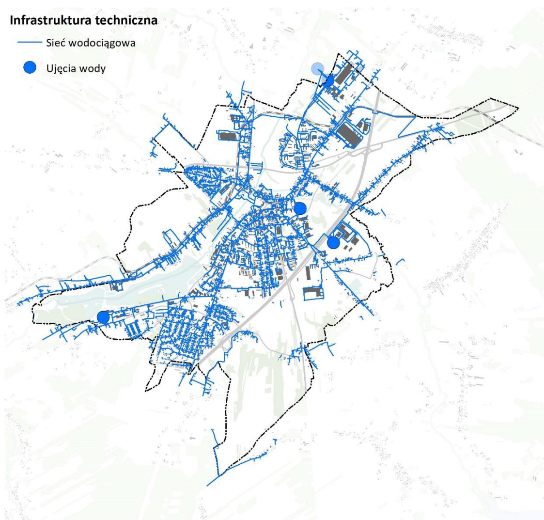
Rysunek 15. System sieci wodociągowej w Rawie Mazowieckiej
