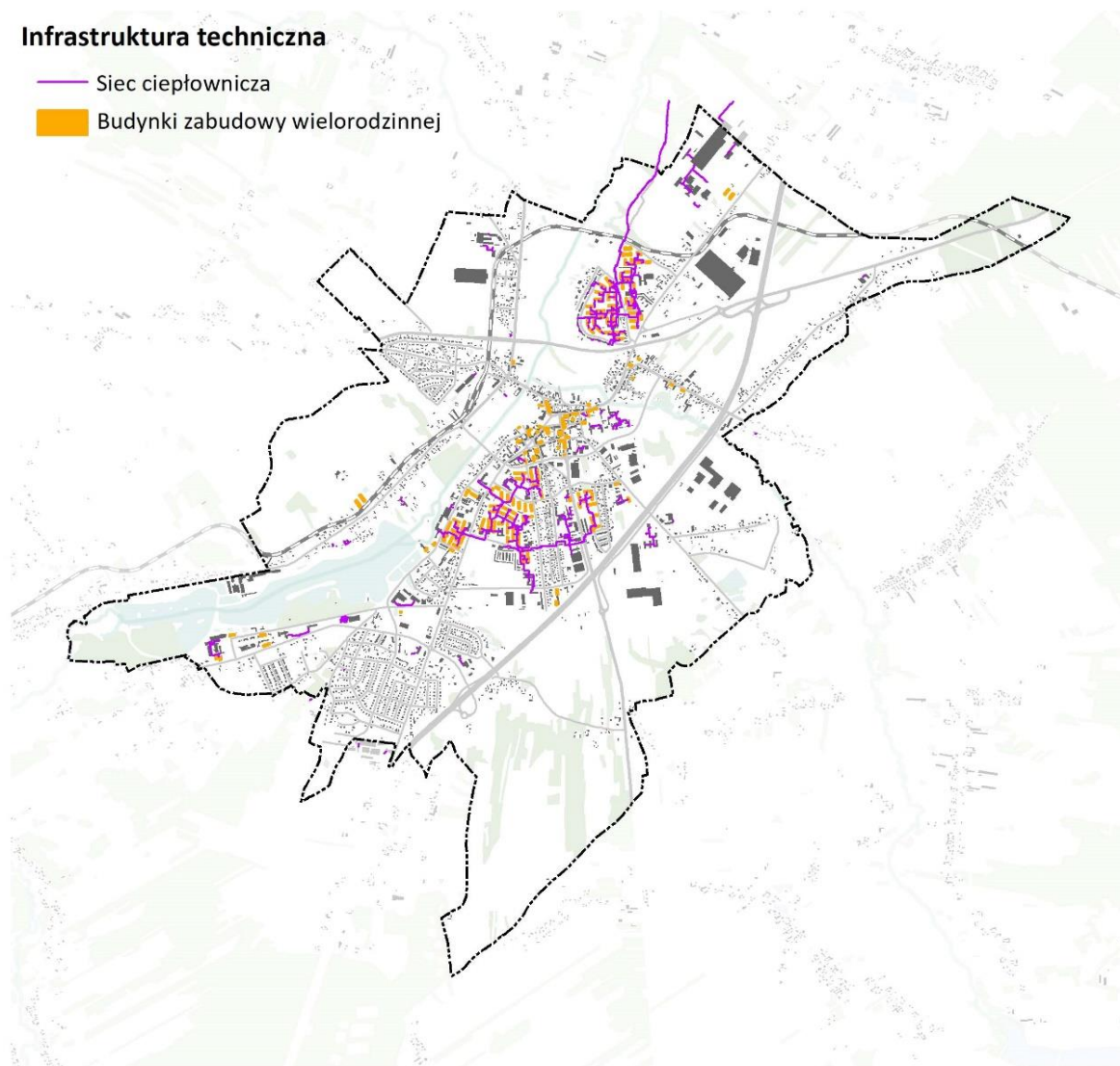
Rysunek 18. System sieci ciepłowniczej w Rawie Mazowieckiej
