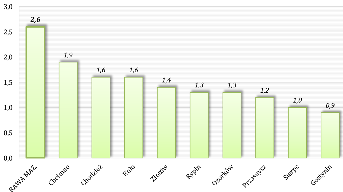
Wykres 1. Średnie stężenie benzo(a)pirenu w powietrzu w 2023 r. [ng/m³] – wartość dla Rawy Mazowieckiej na tle pozostałych miast
